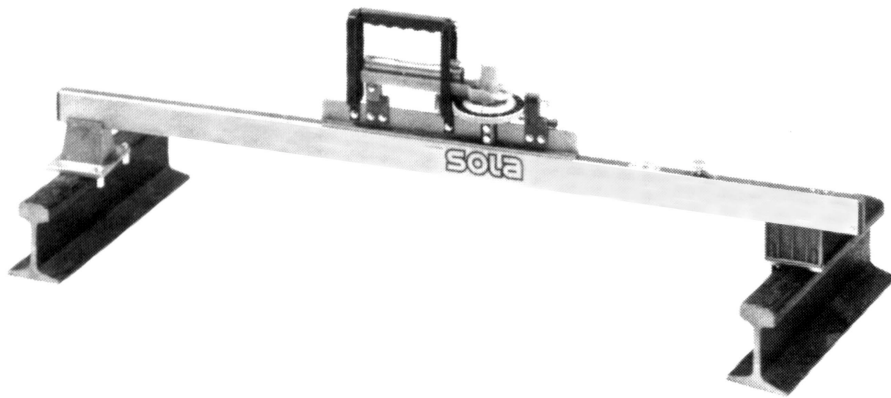
Slika 1: Mjerilo širine i nadvišenja kolosjeka tipa SOLA GW 80
